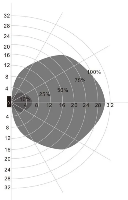
Väggsmonteringsmönster (Enhet: m) Rekommenderad installationshöjd: 1–1,8 m
