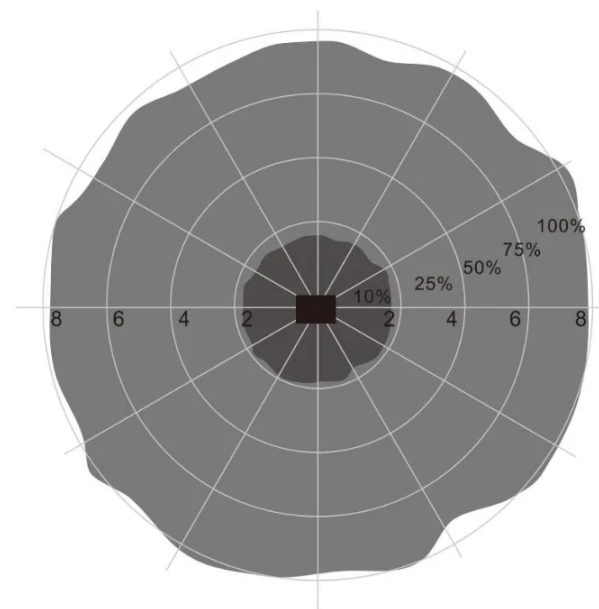
Takmonteringsmönster (Enhet: m) Rekommenderad installationshöjd: 2,5–15 m
